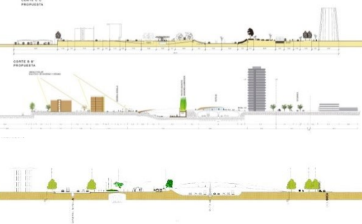
CORTES DE PROPUESTA - DISEÑO URBANO-
